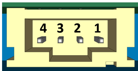
Figura 1b: pin di numerazione della porta di comunicazione VE.Direct, modelli a 75V
