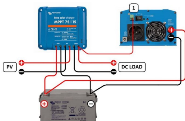
Figura 5: Gli inverter Victron Phoenix 12/800, 24/800, 12/1200 e 24/1200 possono essere controllati connettendo direttamente il connettore di destra (1) del telecomando dell'inverter all'uscita carichi del caricatore solare.
